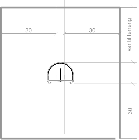
Jernbanetunnel med sikringszone
