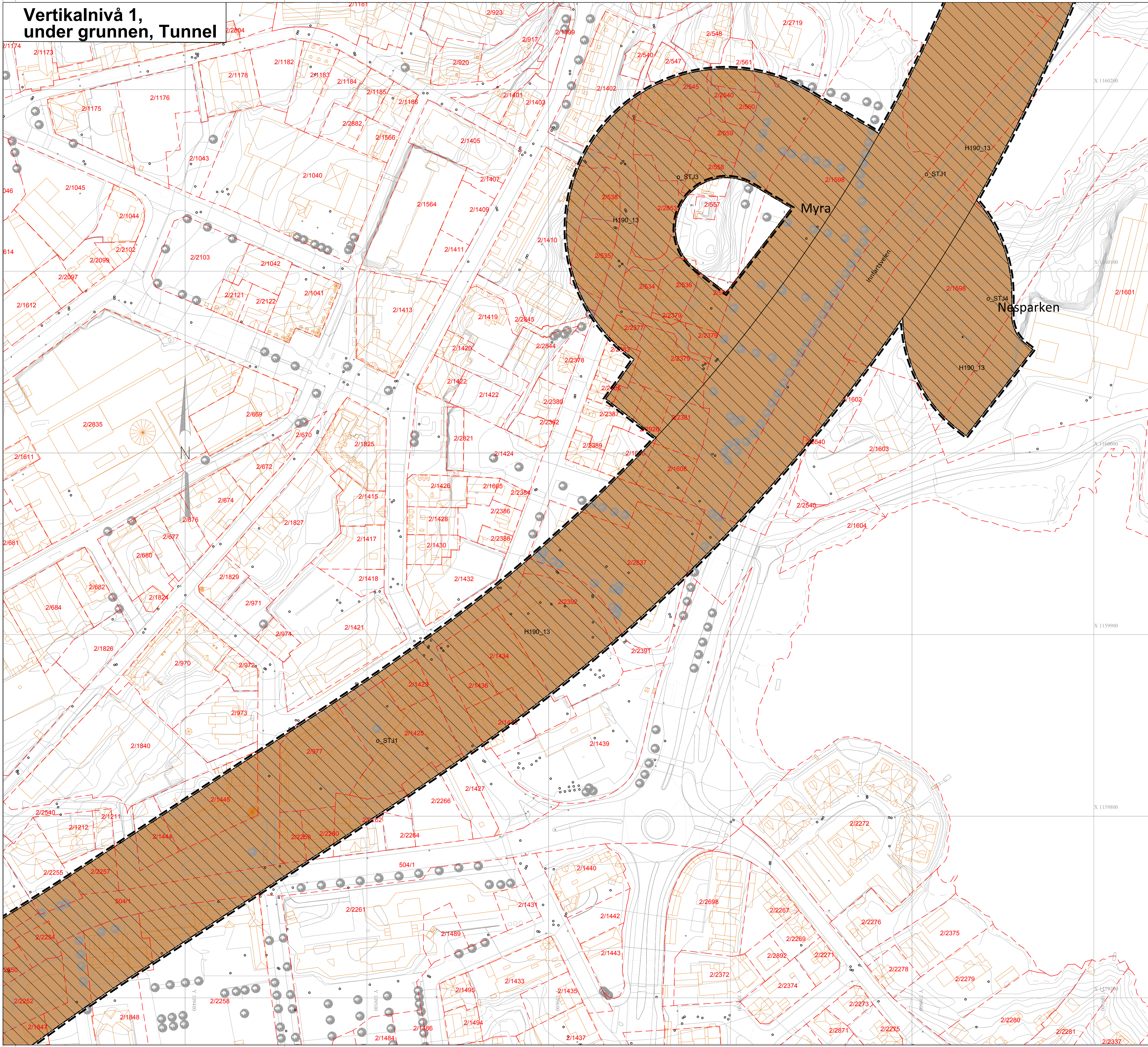
Jernbanetunnel med sikringszone
