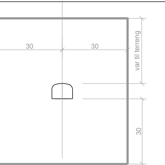
Rømnings tunnel/tverslag med sikringszone 9,5x7m
