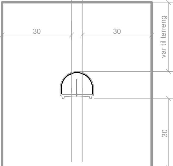
Jernbanetunnel med sikringssone
