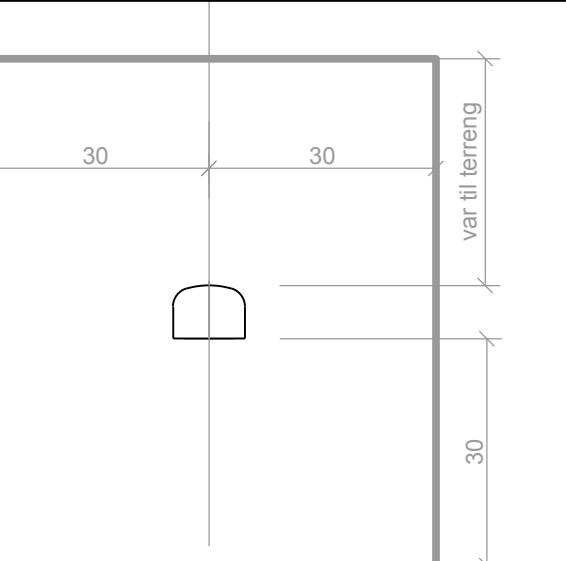
Rømningstunnel/tverrsnitt med sikringssone 9,5x7m
