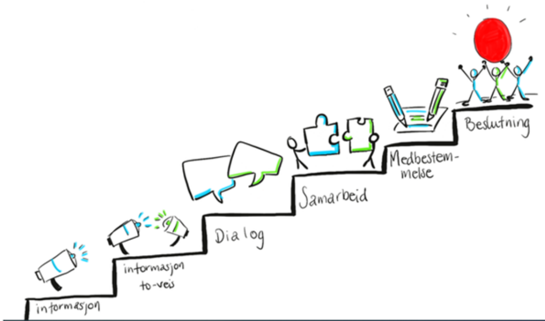
Illustrasjon: Medvirkningstrappa 13
