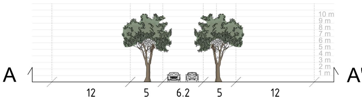
Figur 18 Landskapsskisse som viser tverrsnittet. Kilde: COWI AS, 2019.
