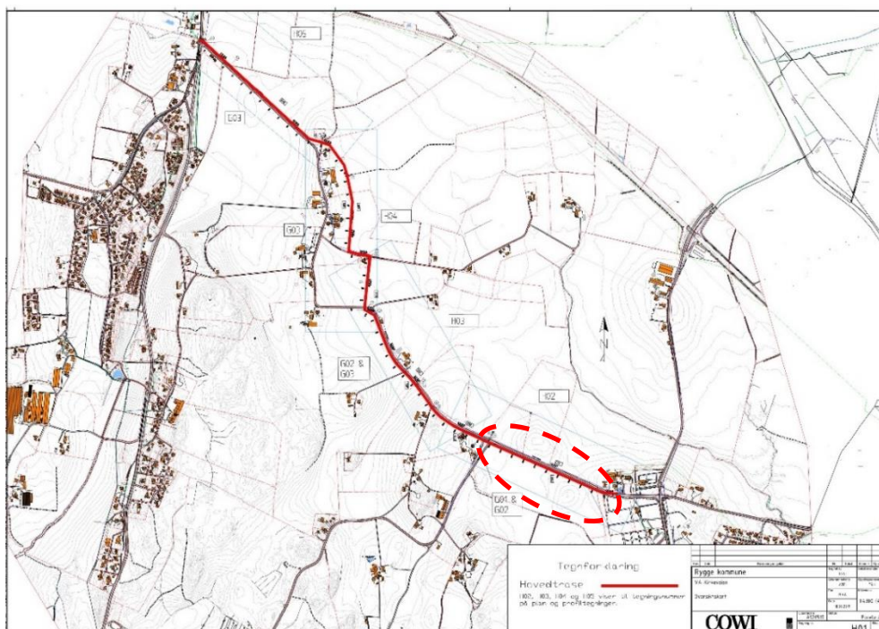
Figur 23 Oversiktskart som viser prosjektert ny hovedtrasé. Planområdet sees til venstre. Kilde: COWI AS, 2019.
