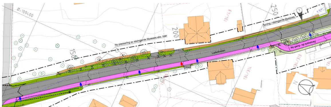
Figur 20 Plantegning av strekningen hvor steingjerdet flyttes og kjøreveien forskyves mot øst. Reetablert steingjerde er vist med lysebrun skravur.
