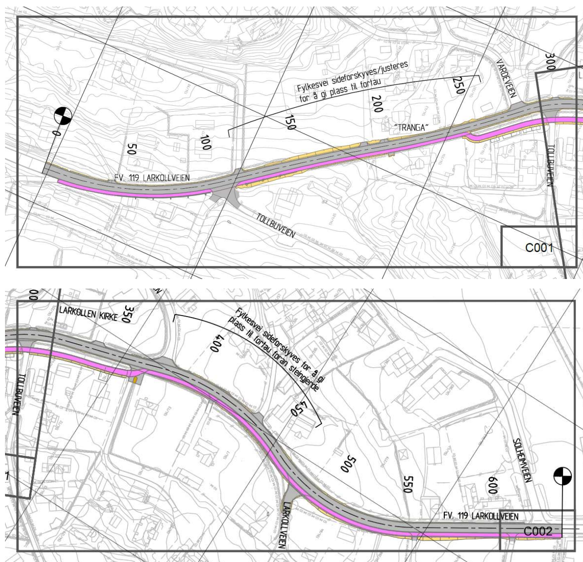
Figur 17 Tegningene viser de planlagte veiløsningene på strekningen. Fortau og gang- og sykkelvei er vist i rosa.
