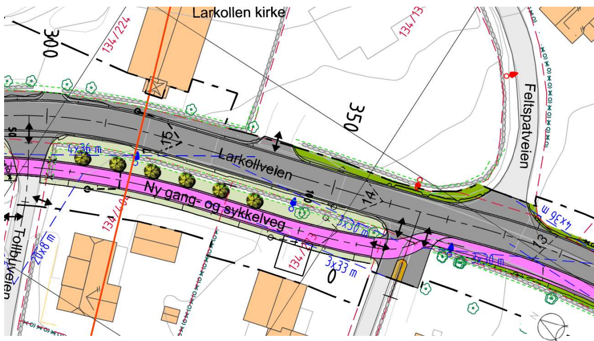
Figur 29 Plantegning av gang- og sykkelveien, hvor Tollbuveien 35 får kjøreadkomst til bolig fra sør.
