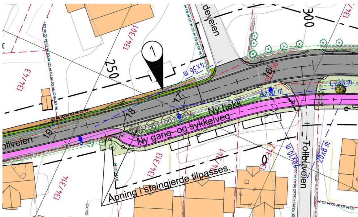
Figur 27 Forslag til plassering av nye biloppstillingsplasser for boligene i Tollbuveien 26, 28 og 30.
