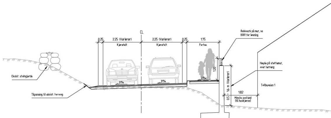
Figur 31 Normalprofil av løsnings ved Tollbuveien 1. Fortauet har her bredde 1,75 meter, som er gjennomgående fortausbredde nord for strekningen med gang- og sykkelvei.
